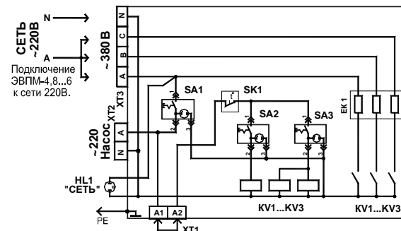
Рис. 8 ЭВПМ-4,8...12(Зреле-3ТЭН). Схема электрическая принципиальная.
