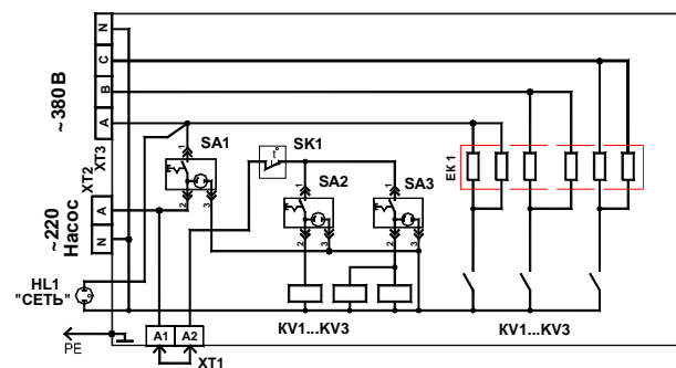
Рис. 9 ЭВПМ-9...12(Зреле-6ТЭН). Схема электрическая принципиальная.
